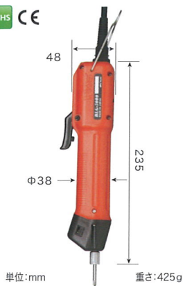
単位:mm 重さ:425g
